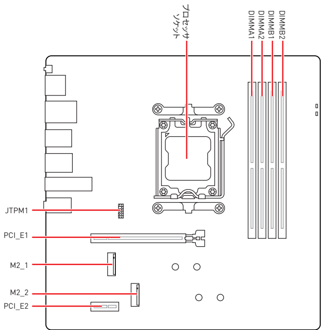
上面図
